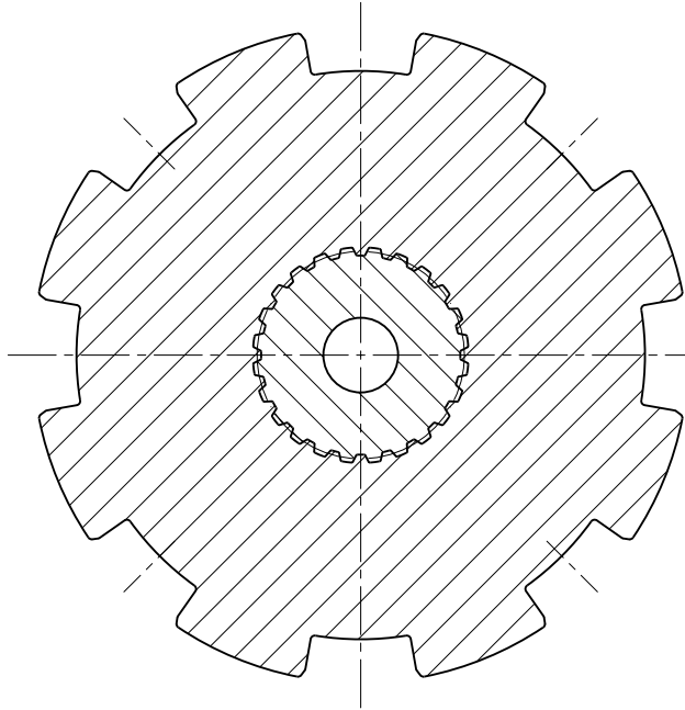
Е-Е (1:1)
