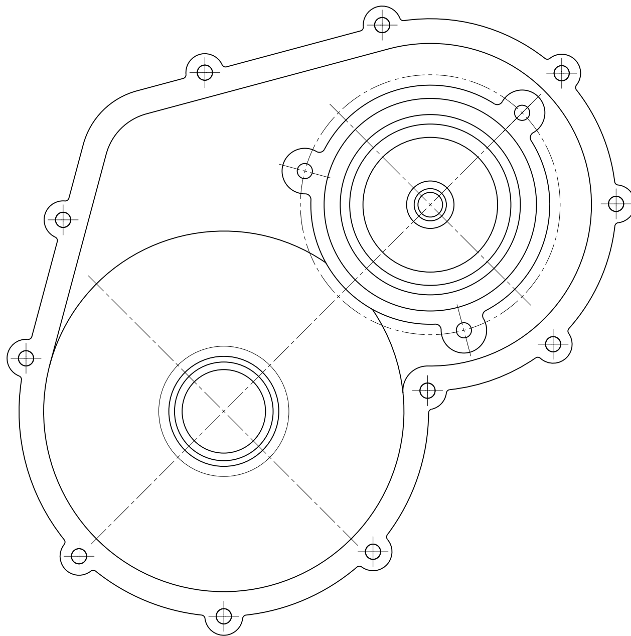
Г-Г
